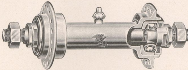
Modell No. 90 - Vorderrad-Nabe
