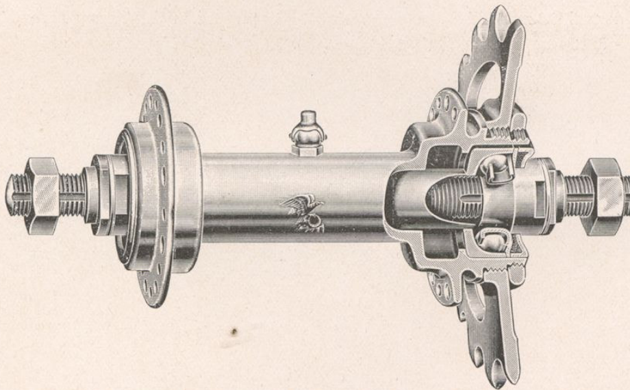
Modell No. 91 - Hinterrad-Nabe mit Raum für Kettenkasten
