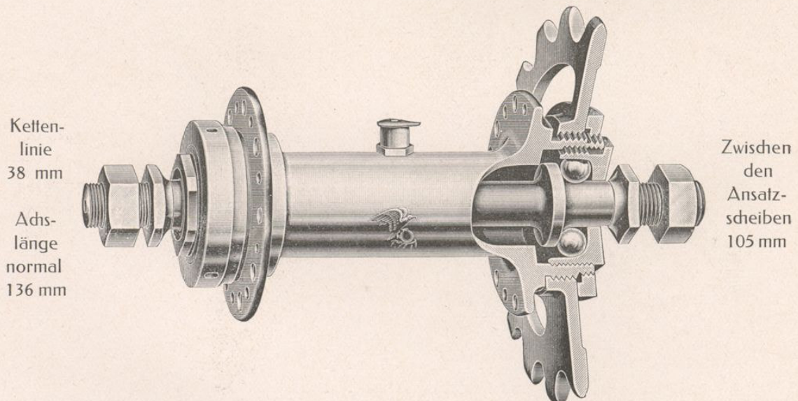
Modell No. 61 - Hinterrad-Nabe
