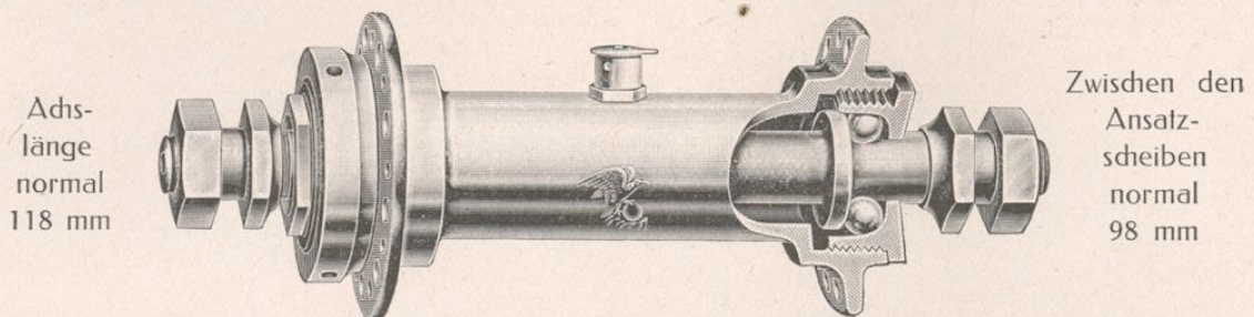
Modell No. 60 - Vorderrad-Nabe
