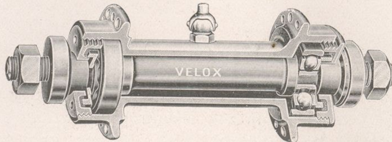
Modell No. 400 · Velox-Vorderrad-Nabe (gesetzl. geschützt)
