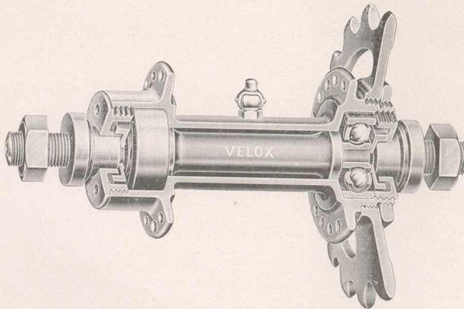
Modell No. 401 · Velox-Hinterrad-Nabe (gesetzl. geschützt)
