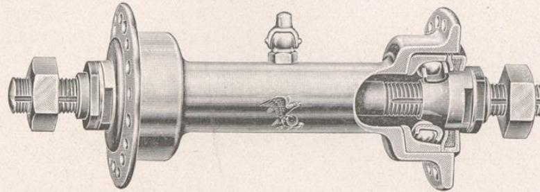
Modell No. 80 - Vorderrad-Nabe
