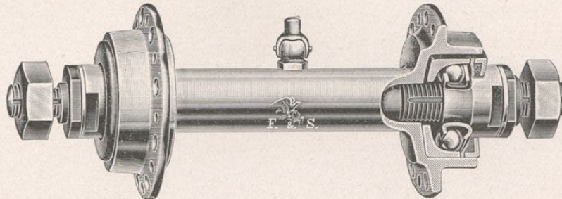
Modell No. 40 Vorderrad-Nabe H
